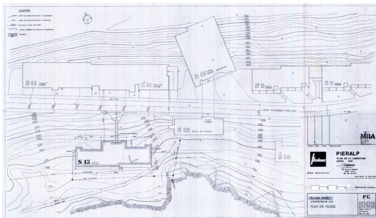
Plan de masse. M.B. A architectes, 17 août 1984 (AC Arâches-la-Frasse)
