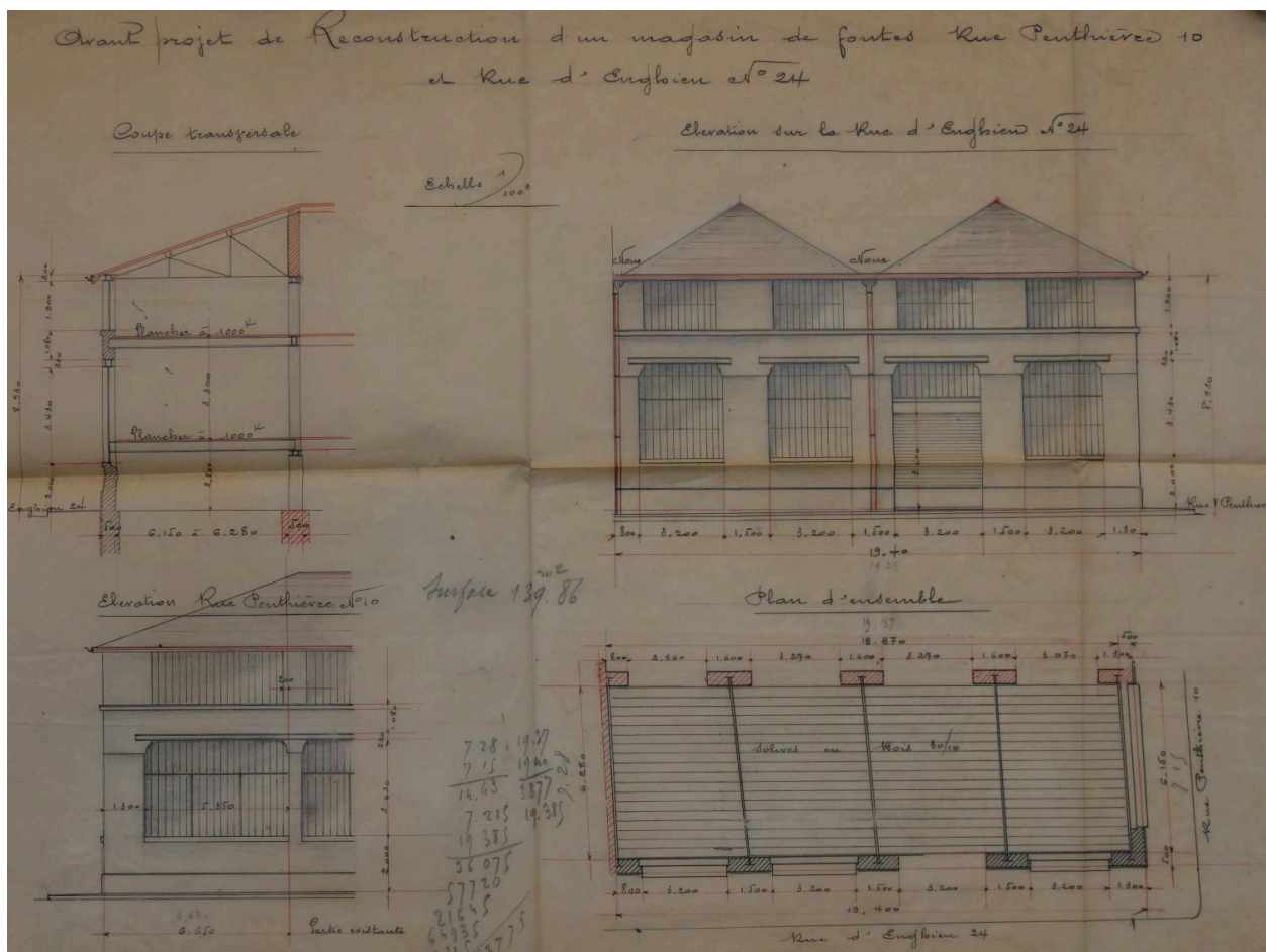
Plan de reconstruction du magasin des fontes, usine Descours & Cabaud 1903, Lyon 2e (ACL314W191-507)
