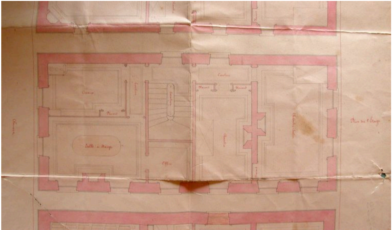
Plan du premier étage du bâtiment. Plan dressé par Stéphane Boulin, architecte départemental, 1878.
