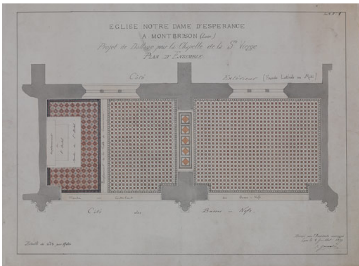
Eglise Notre-Dame d'Espérance à Montbrison. (Loire). Projet de dallage pour la chapelle de la Ste Vierge. Plan d'ensemble. Feuille n°1.
