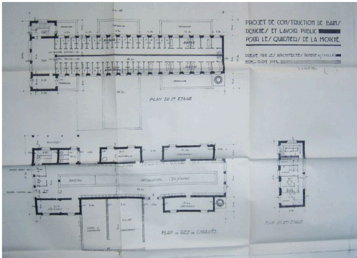
Plan du rez-de-chaussée, 1er étage et 2ème étage. Projet de bains douches lavoir au centre de la cité jardin de la Mouche. A. E. Chollat et V. Robert architectes, 11 avril 1930. Ech. 1 : 100 (Arch. mun. Lyon)
