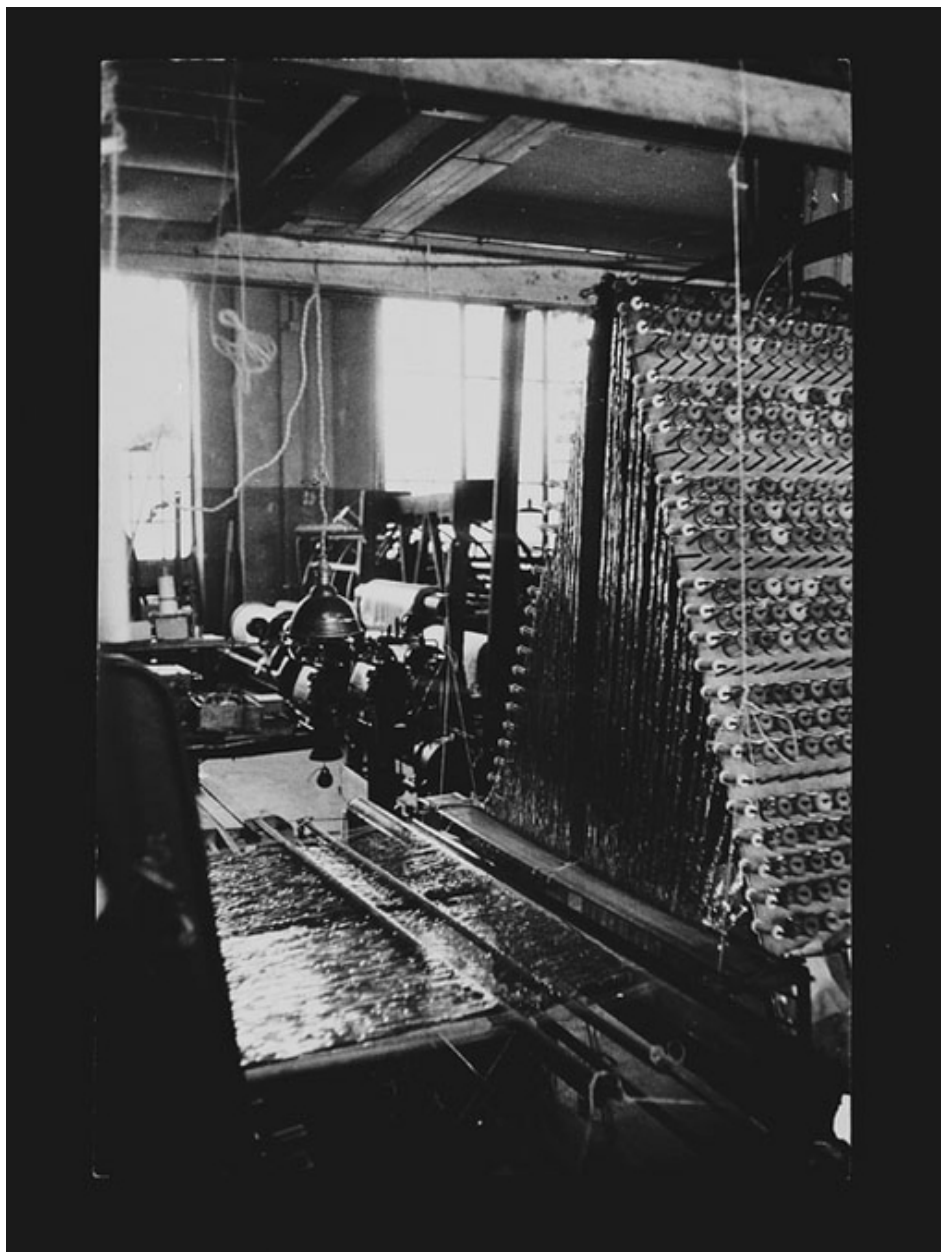
Métier jacquard n° 7, cantre d'alimentation, mouvement taffetas, photo prise en 1960, archives privées DLMI
