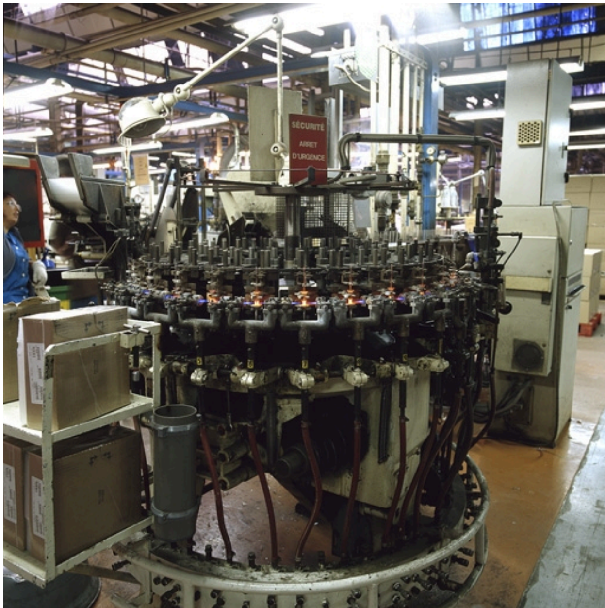
Vue d'ensemble de la machine des filament
