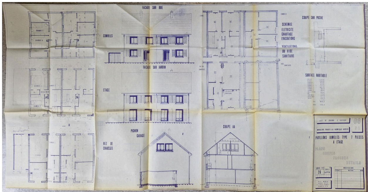
Projet du lotissement : plans, coupes et élévations des pavillons jumelés de type F7 à étage, 1972.
