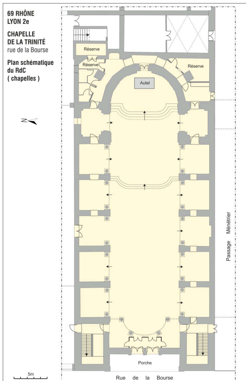
Plan schématique, rez-de-chausée (état actuel). Dess. A. Céréza
