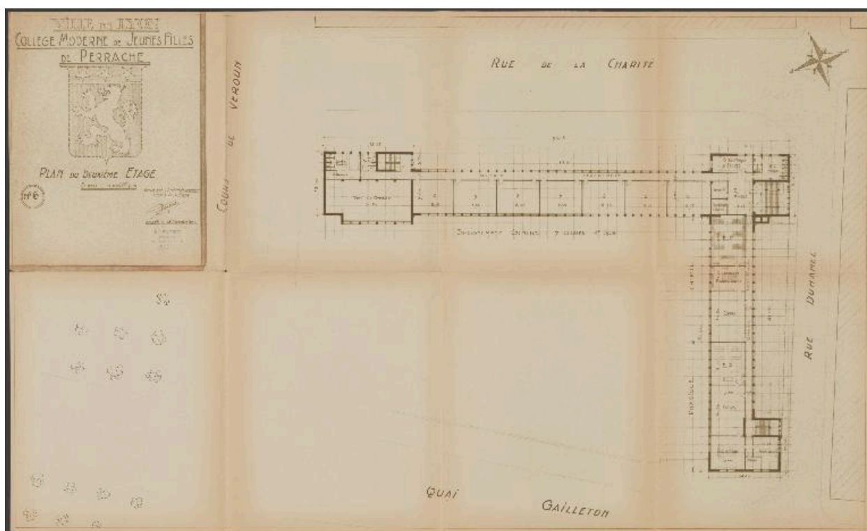
Plan du 2e étage, par E. Payen, 1954 (AC Lyon, 838 WP 001)
