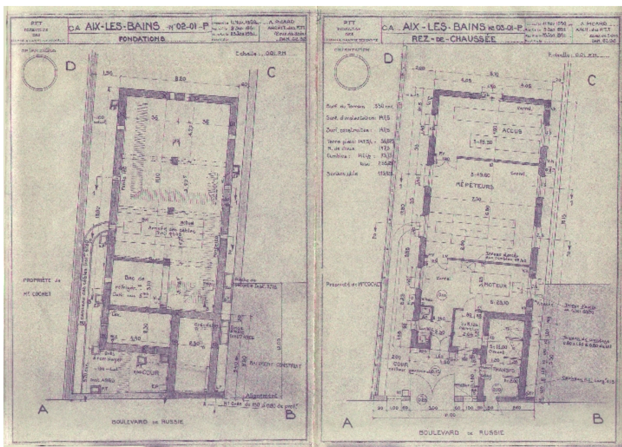
Plans des fondations et du rez-de-chaussée
