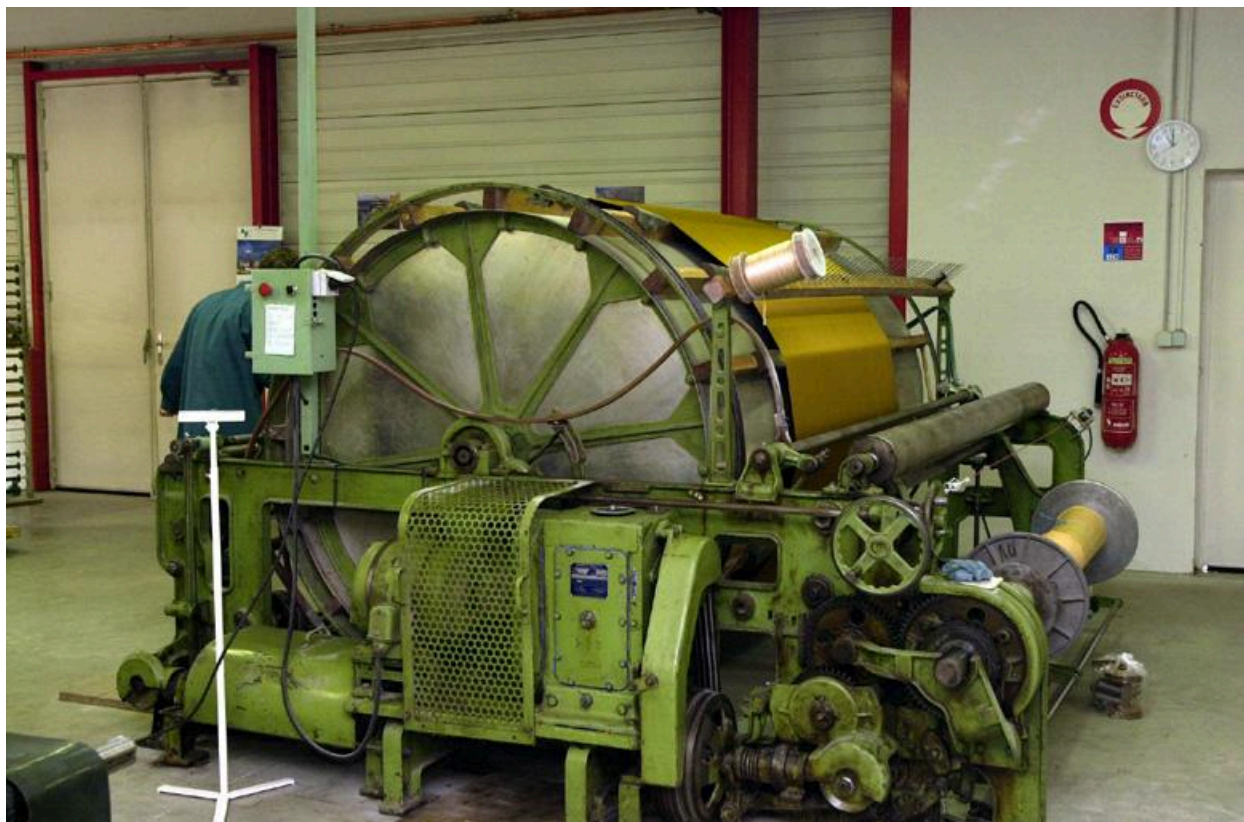
Ourdissoir horizontal
