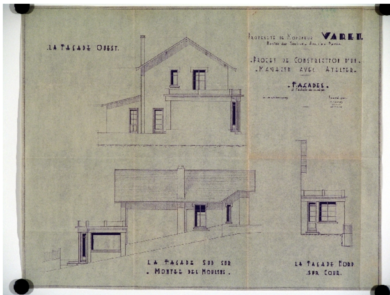
Projet de construction : façades
