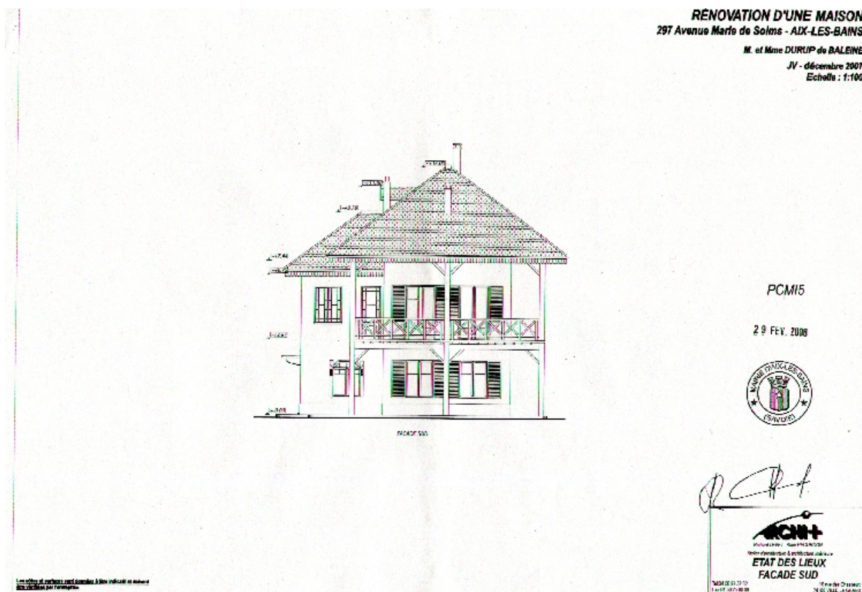
Elévation sud
