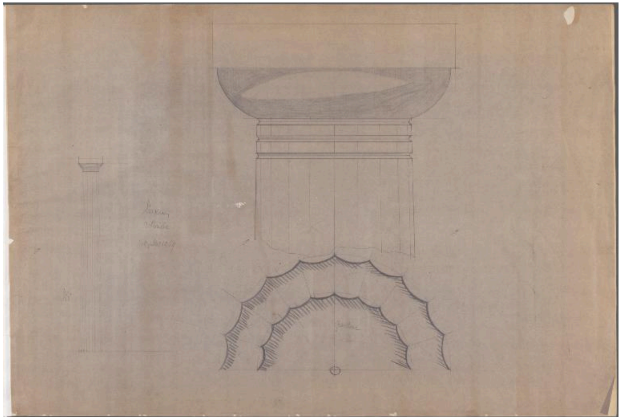
Musée Guimet, rotonde, colonnes : plan, élévation et détail du chapiteau, 9 juillet 1969. AC Lyon, 1480 WP 361 M
