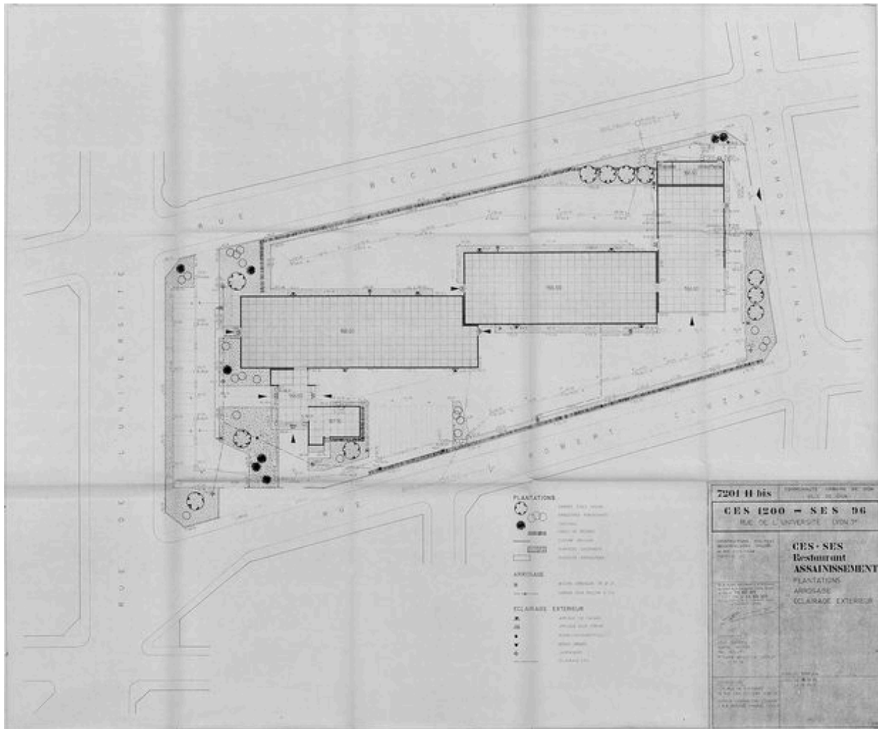
Plan de situation (Arch. dép. Rhône, 686 W 130, tirage d'architecte, 1972).
