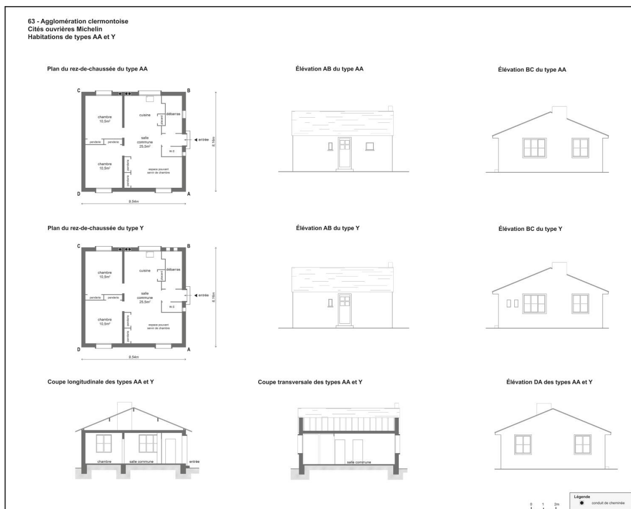
Plans, coupes, façades des habitations de types AA et Y
