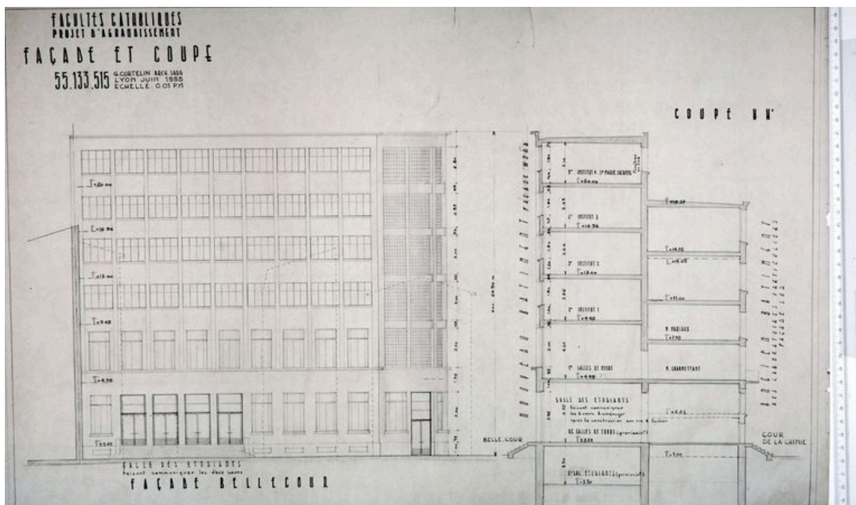
Plan, projet de façade et coupe du bâtiment ISARA 1ère tranche par G. Curtelin, 1956
