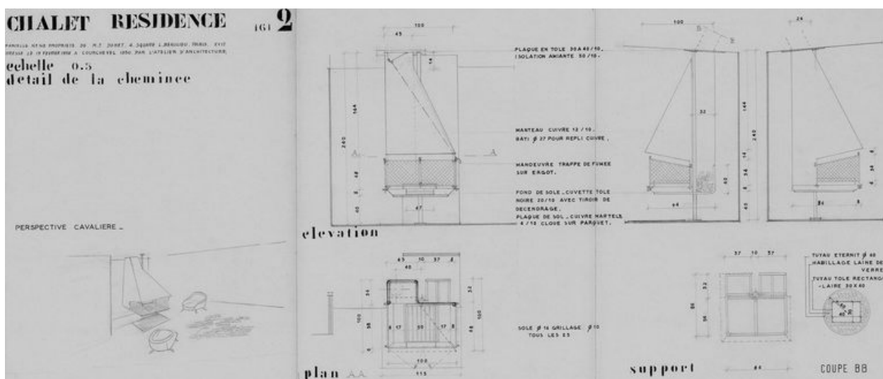
Chalet résidence. Détail de la cheminée. Atelier d'Architecture de Courchevel, 19 février 1958 (AD Savoie. 6J 172)
