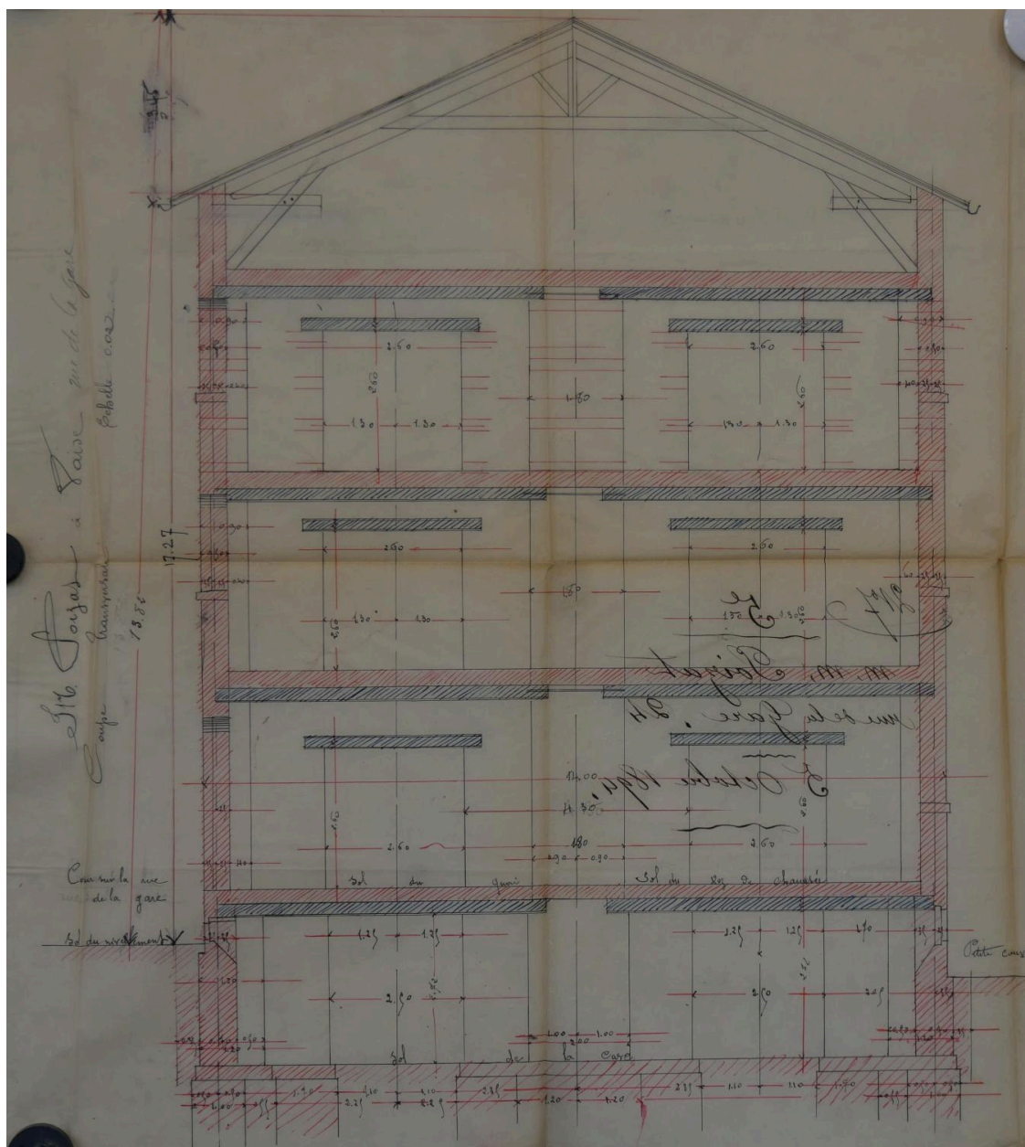
Plan usine Poizat 1894, coupe (ACL : 314W93 - 217)
