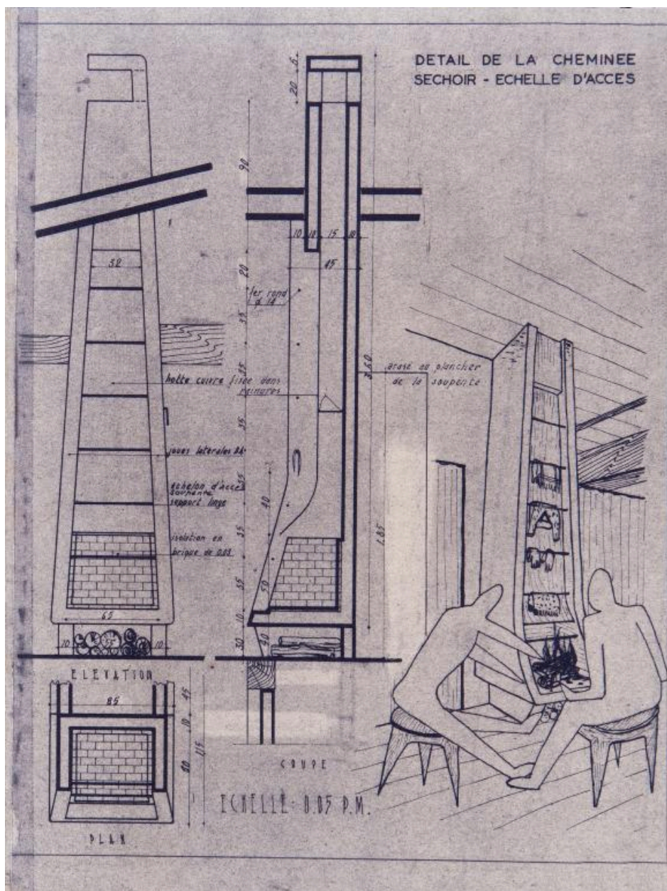
Chalet Intimité : détail de la cheminée, 1955
