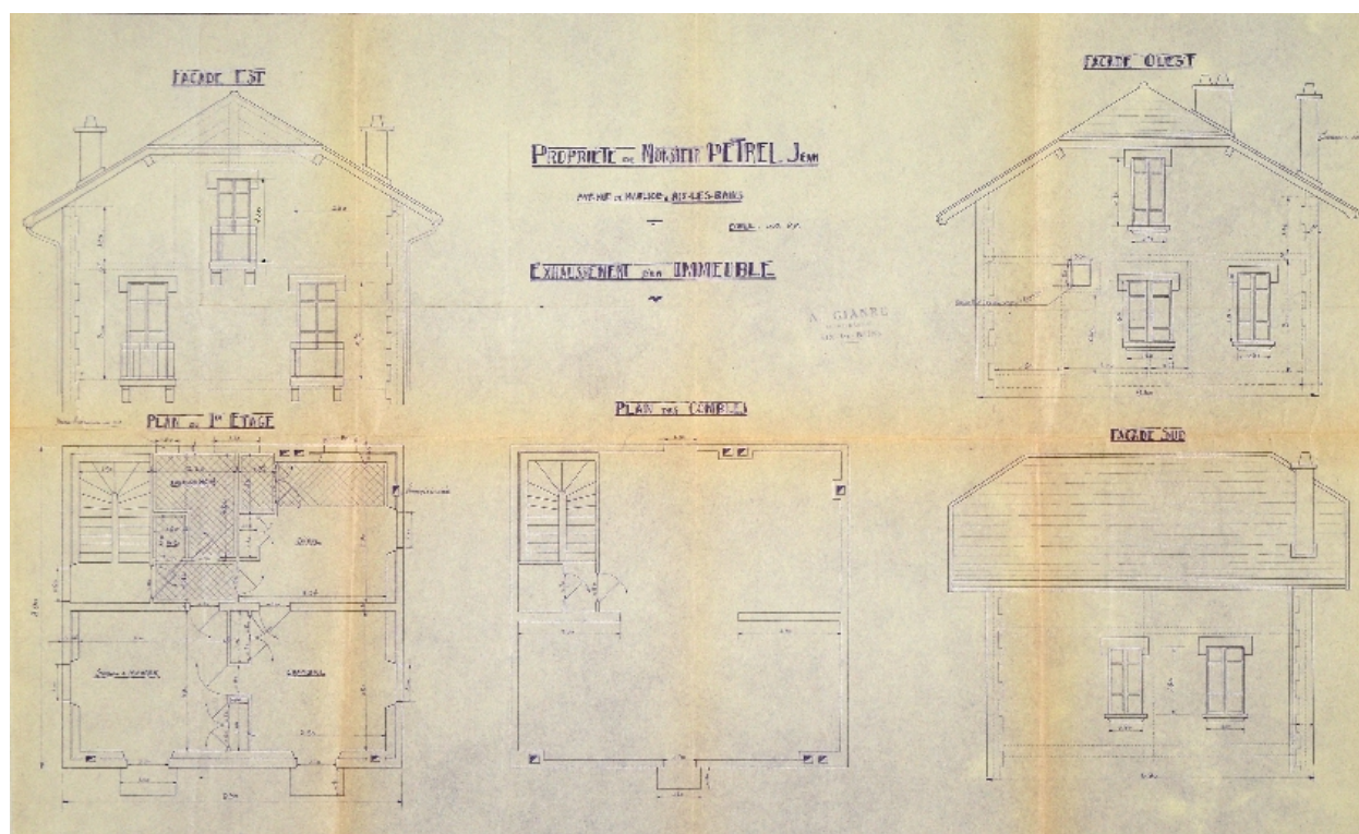
Exhaussement de 1923 : plans et élévations
