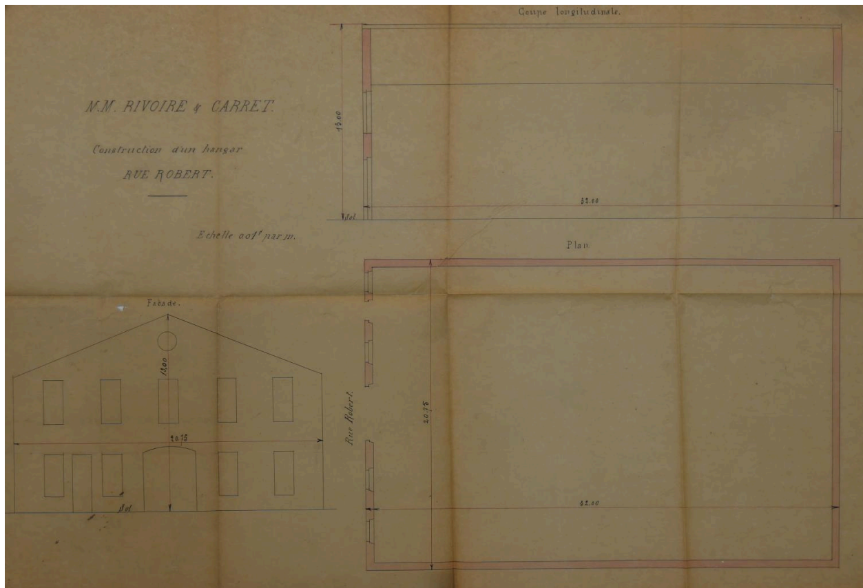
Plans ancienne usine Rivoire et Carret en 1885, site rue Robert Lyon 3e arr. (ACL 314w10-207)
