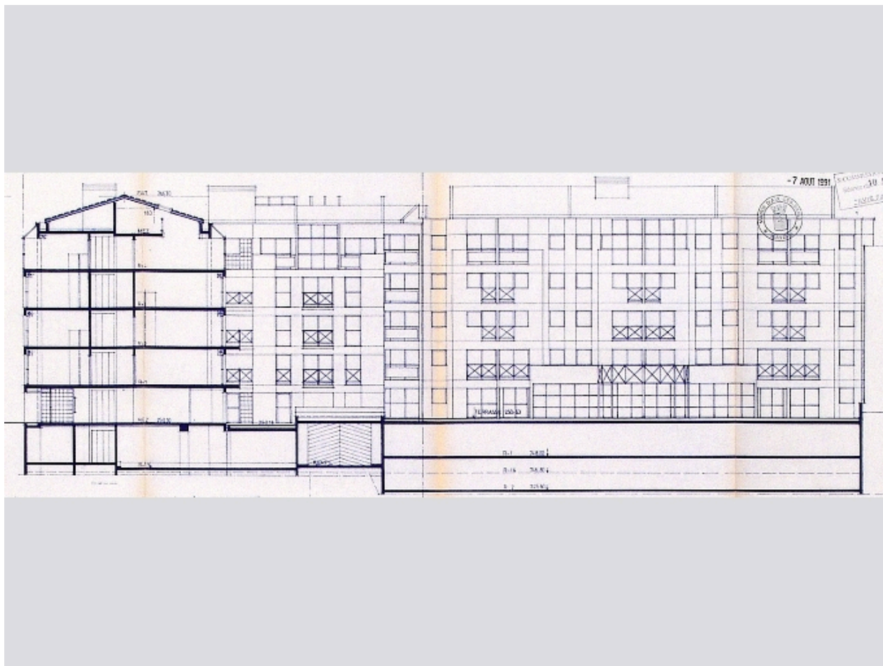
Coupe nord-sud
