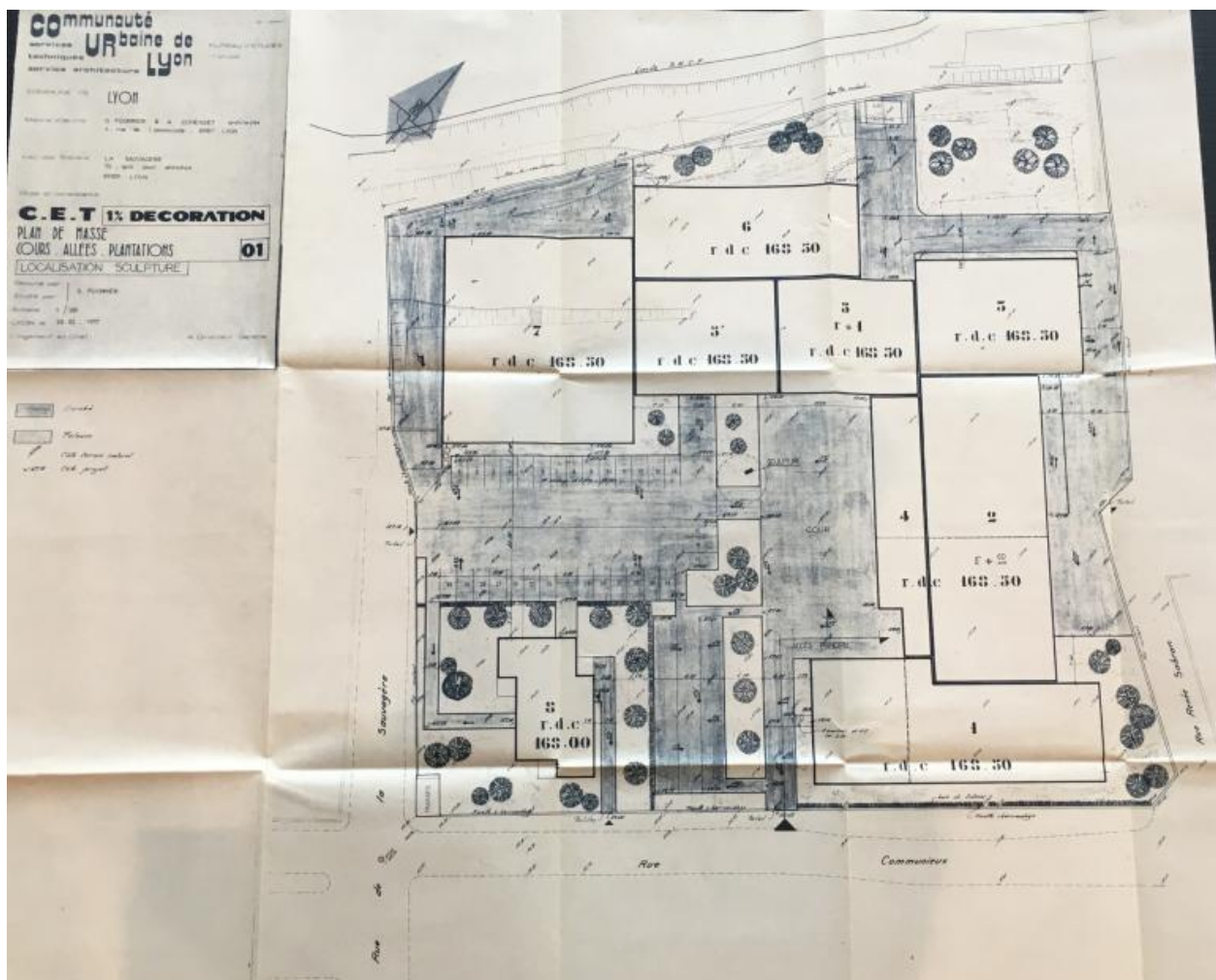
Plan d'implantation de l'œuvre (Fourrier, 1977) (AN 19880466/126)
