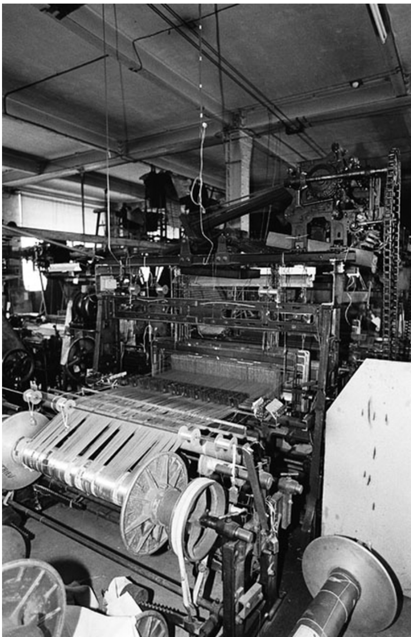
Vue d'ensemble du métier jacquard de marque Bruyère-Banzet SACM, à mécanique ratière
