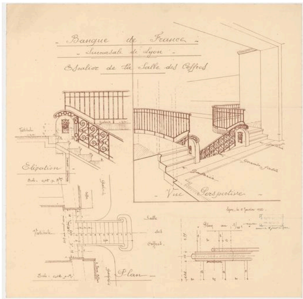
Dessin du nouvel escalier (1922) descendant à la salle des coffres (Banque de France, service du Patrimoine Historique et Artistique, non coté, dessin de Xavier Thoubillon).
