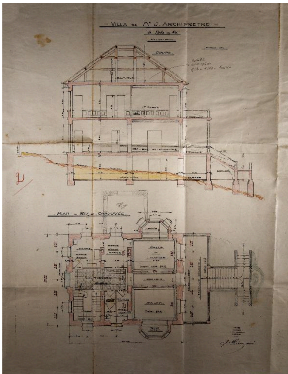
Coupe et plan du rez-de-chaussée, 1926
