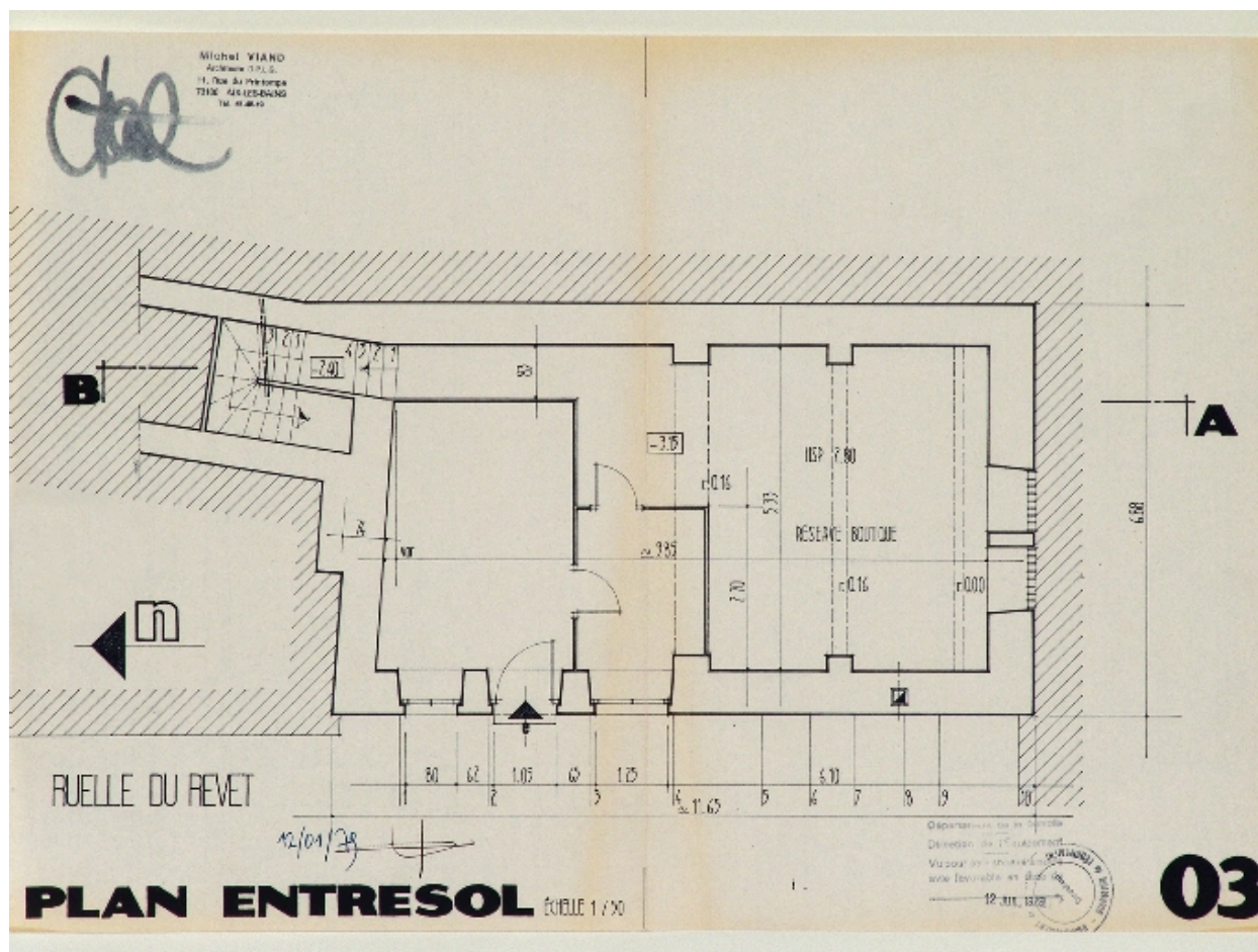
Plan de l'entresol
