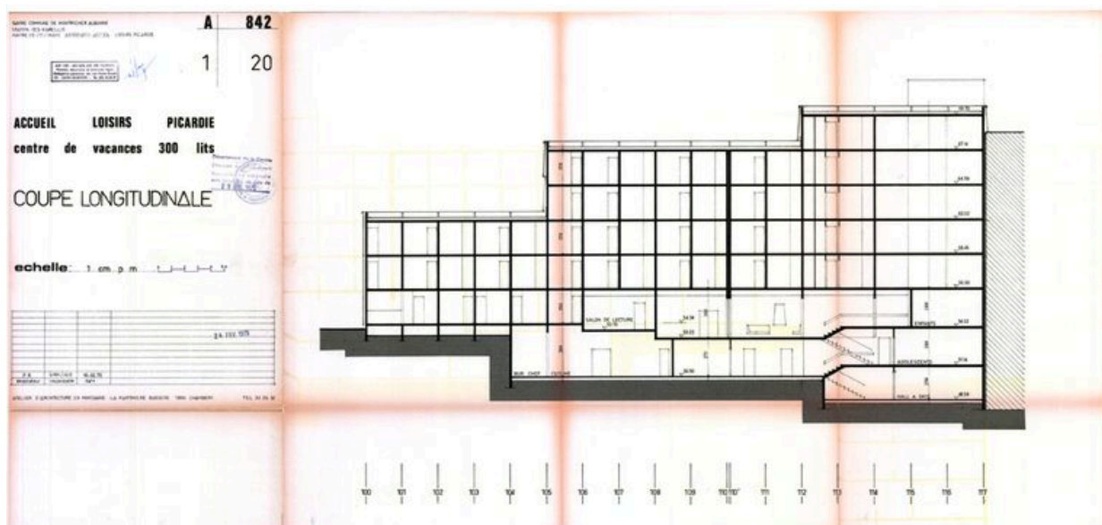
Accueil Loisirs Picardie. Coupe longitudinale / Atelier d'Architecture en Montagne, 10 février 1975 (AC Montricher-Albanne)
