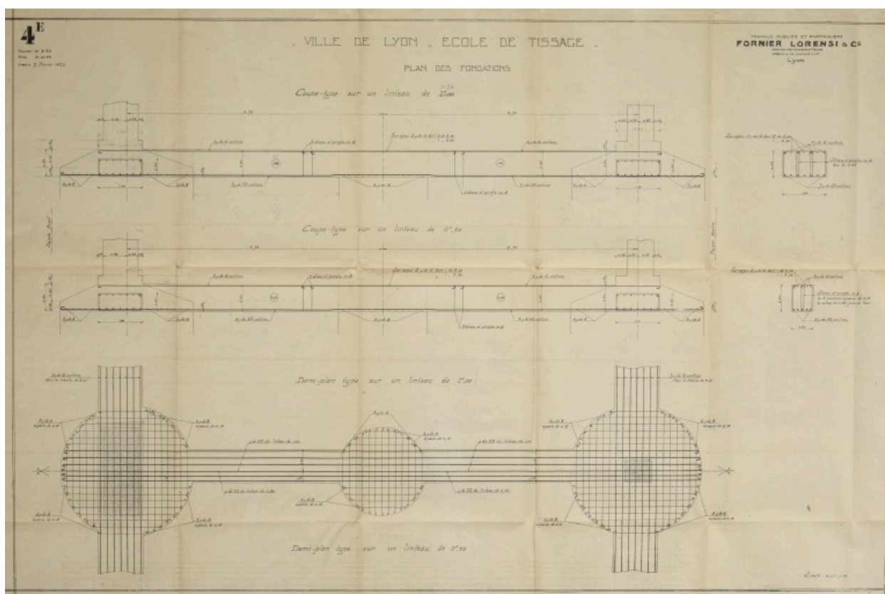
Ecole de tissage, plan des fondations. 7 février 1929. Fornier et Lorensi & Cie, ingénieurs constructeurs. (AC Lyon. 511 WP 002)
