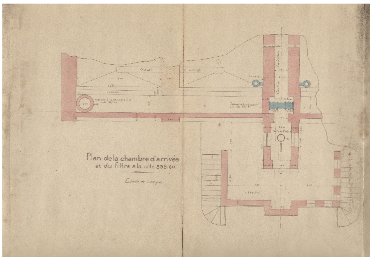
Plan de la chambre d'arrivée
