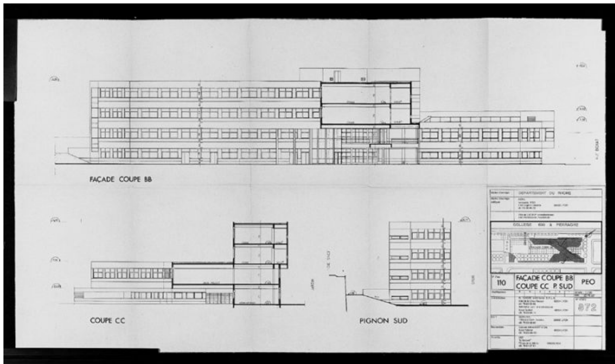
Façade et coupe BB, coupe CC, pignon sud
