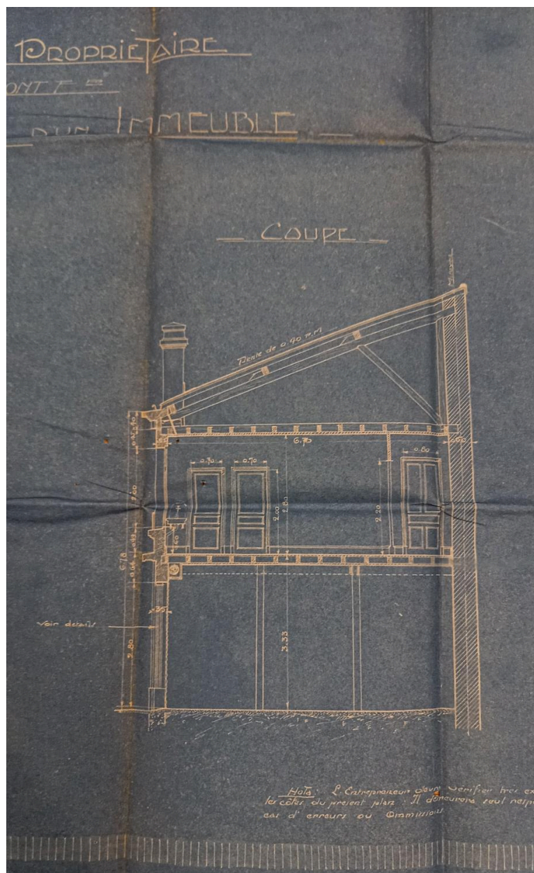
Coupe du 21 avenue d'Italie (fond de parcelle)
