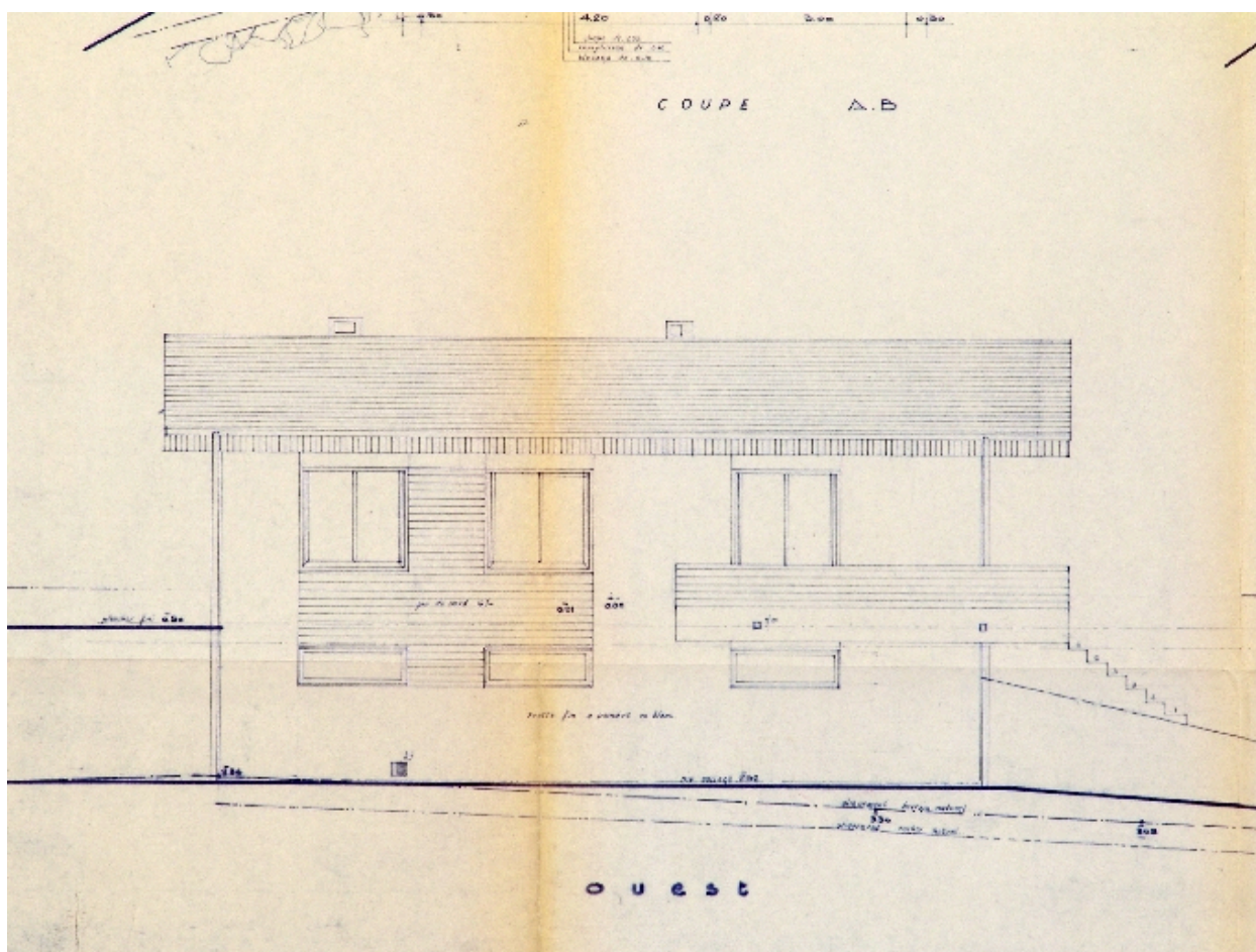
Elévation ouest
