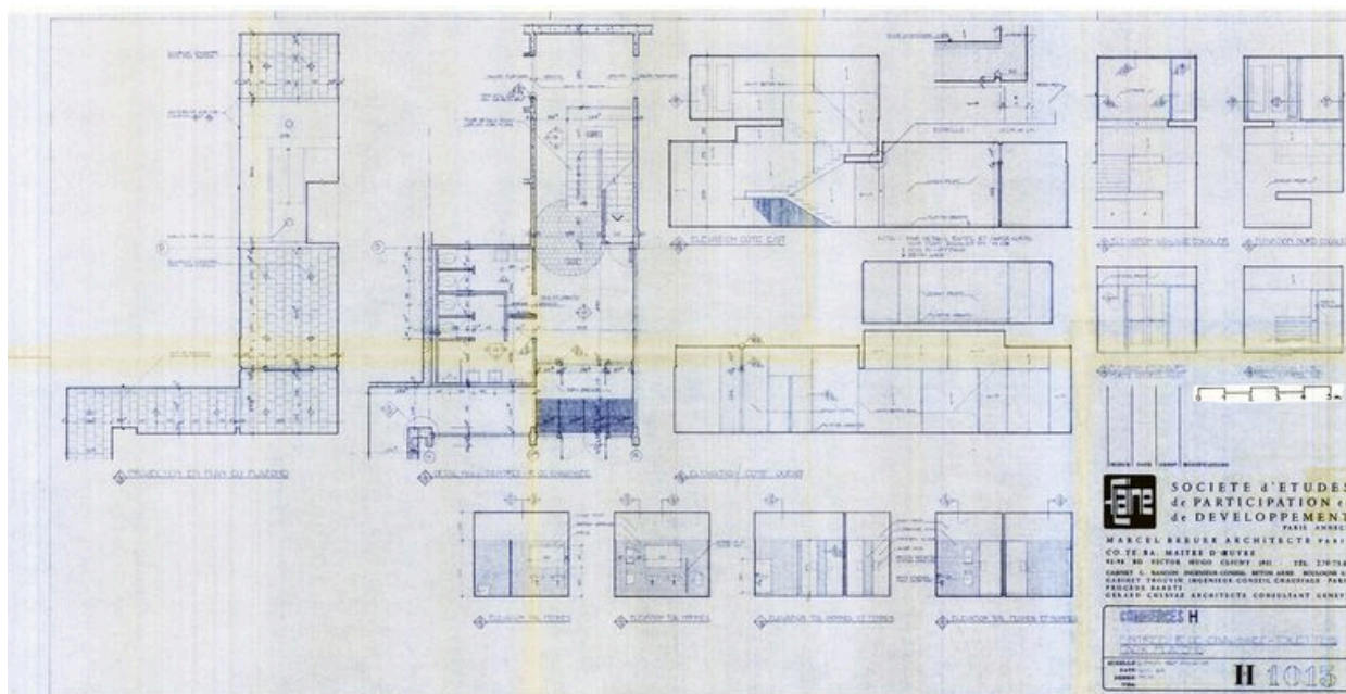
Commerces H. Plan, élévations, détails. Rez-de-chaussée, entrée, toilettes, faux-plafond. Marcel Breuer architecte, 16 janvier 1967 (AC Arâches-la-Frasse)
