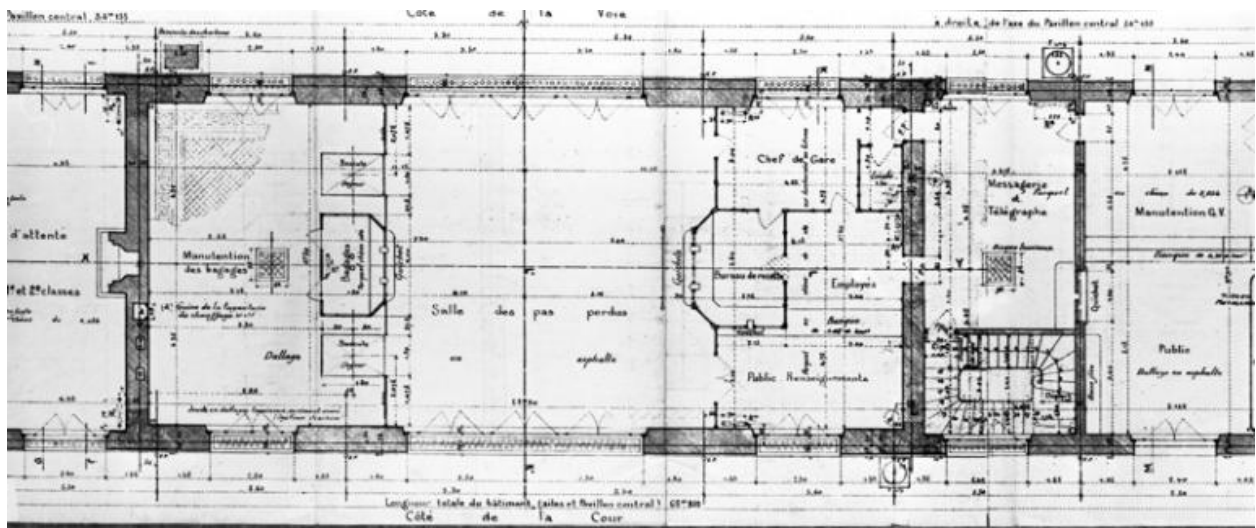
Gare de Châtel-Guyon. Bâtiment des voyageurs. Plan du rez-de-chaussée.
