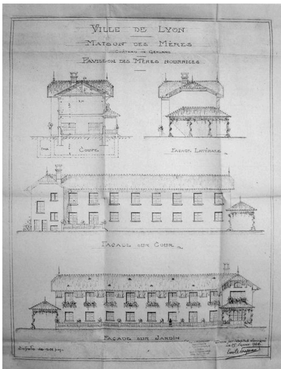
Pavillon des mères nourrices, façades, Emile Poignant, 1924 (AC Lyon 1741 W 5)
