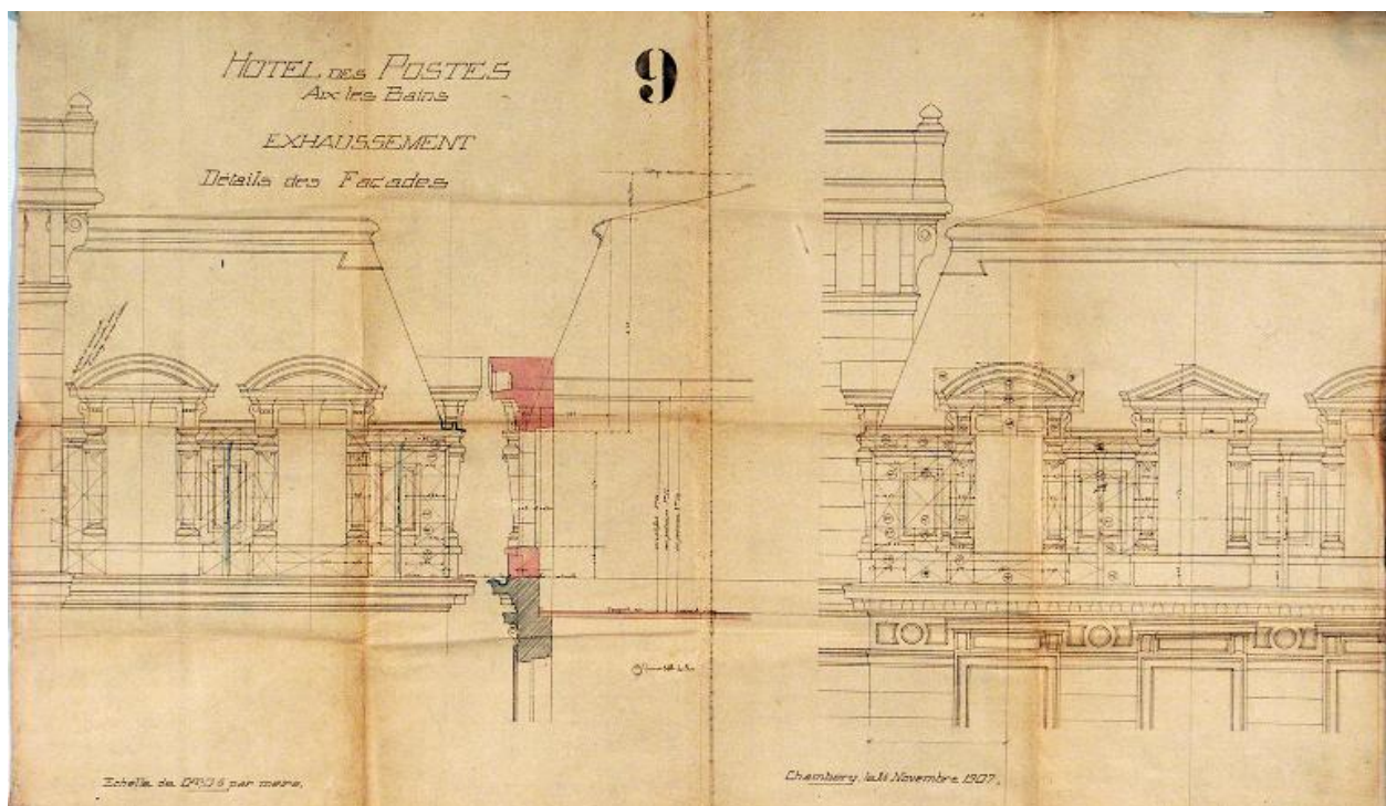
Exhaussement, 1907 : détails des façades
