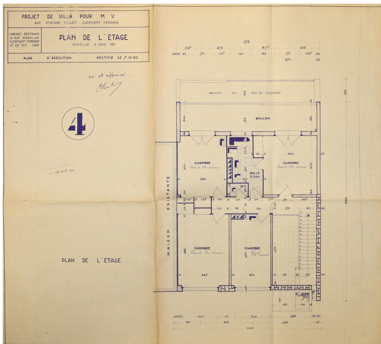
Clermont-Ferrand, la maison V., plan de l'étage, Cabinet Bertrand - Jean-Paul Bertrand architecte, octobre 1960 (archives municipales de Clermont-Ferrand).
