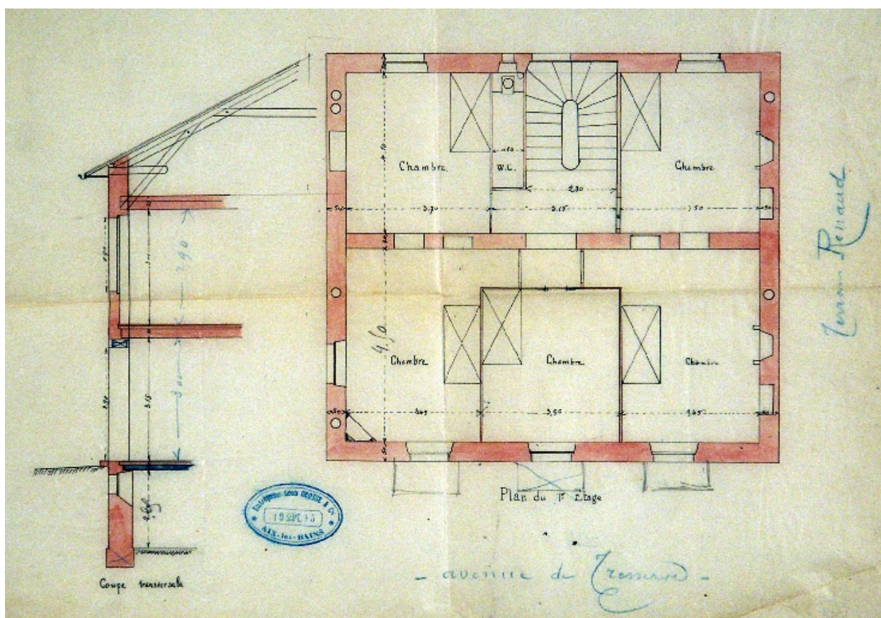
Plan du 1er étage et coupe
