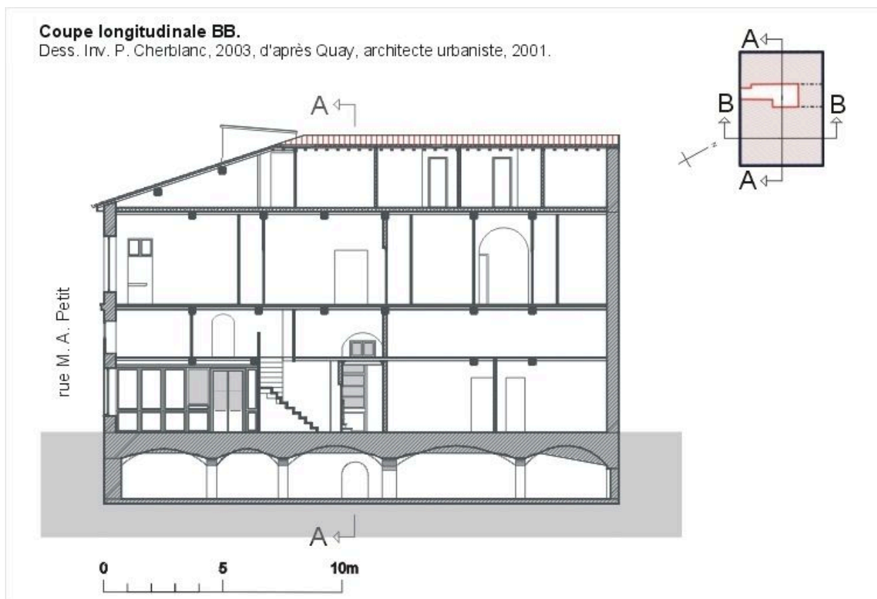
Coupe longitudinale
