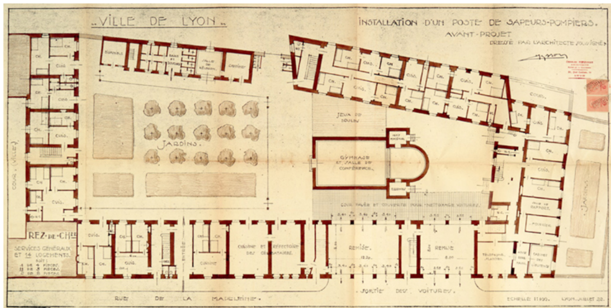
Installation d'un poste de sapeurs-pompiers. Avant-projet, par Charles Meysson, 22 juillet [1922]. Plan du rez-de-chaussée. 1 : 100 (AC Lyon. 0470 WP 026)
