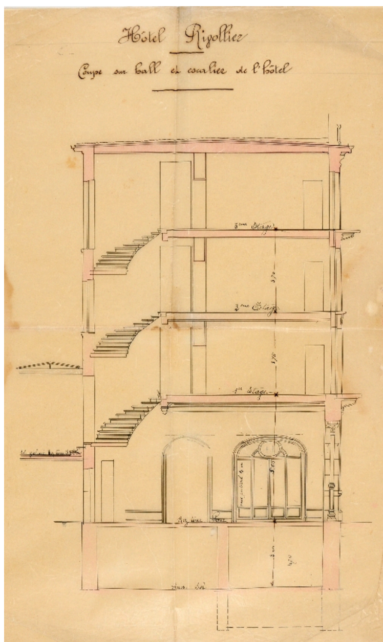
Coupe sur le hall de l'hôtel
