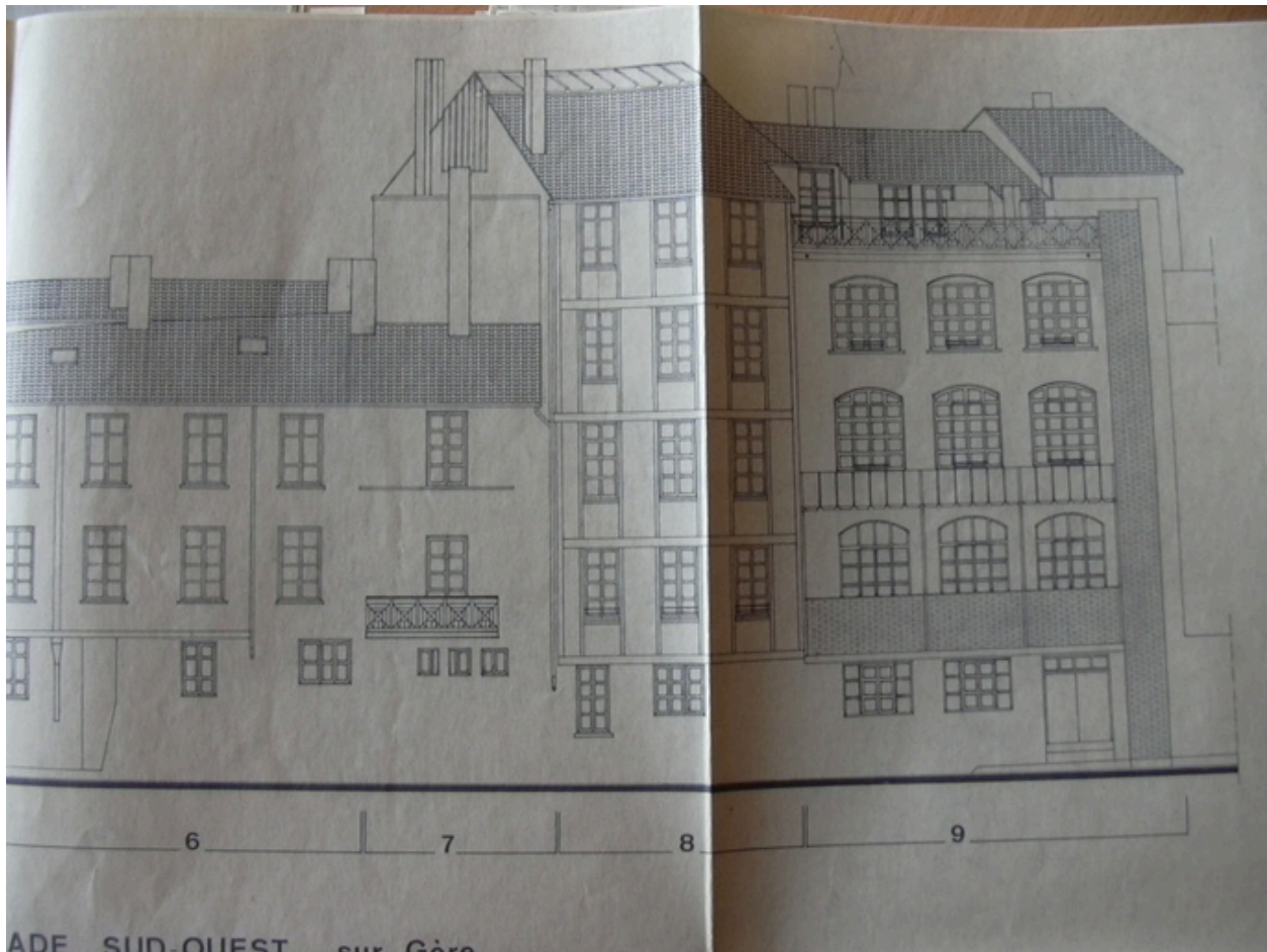
Façade sur Gère, projet 1980 II
