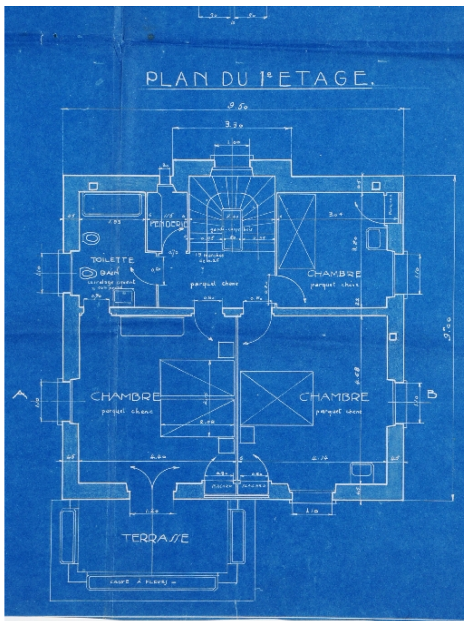
Plan du 1er étage
