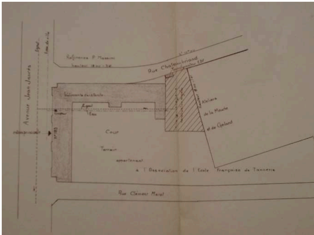
Plan de l'Ecole Française de Tannerie ; Atelier ; Plan d'ensemble avec canalisations
