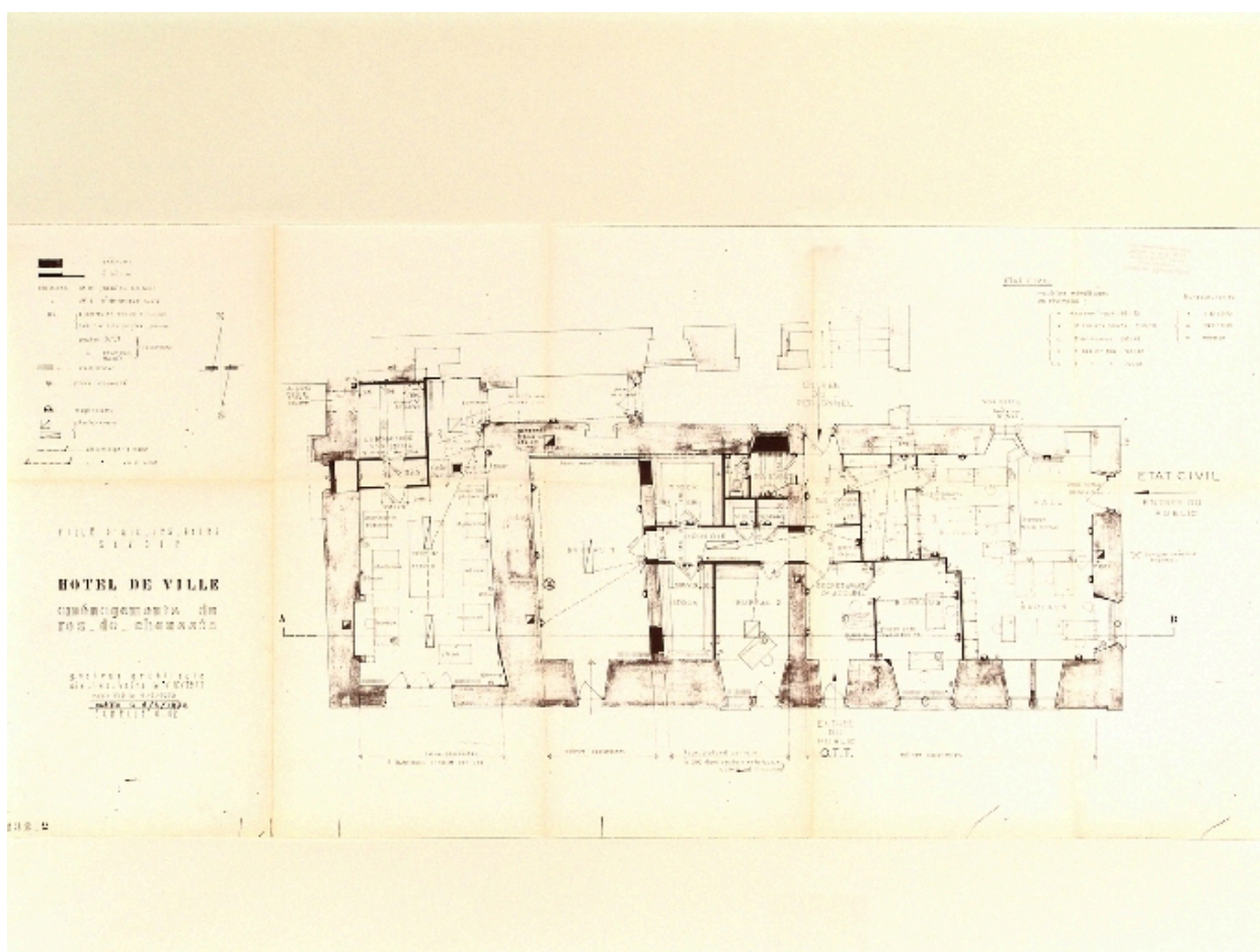
Plan d'aménagement du rez-de-chaussée
