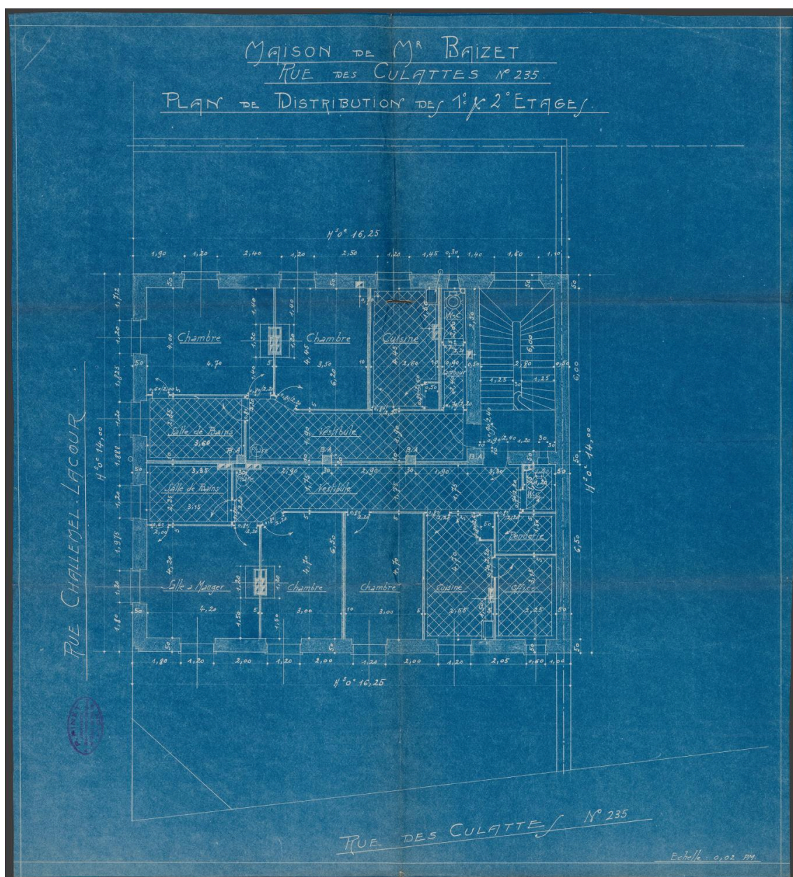
Plan de distribution des 1er et 2e étages
