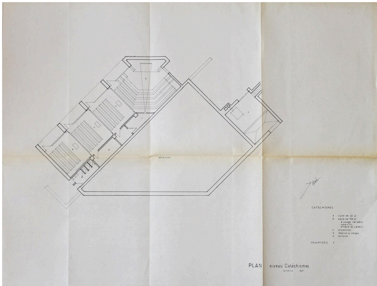
Brioude, chapelle de la Borie Darles, plan du niveau « catéchisme », avant-projet non daté (vers juin 1964), Guy Bion architecte, Archives de la paroisse Saint-Julien de Brioude.
